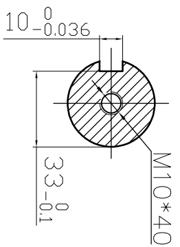
A-A(2:1)
