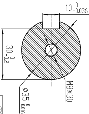
B-B (2:1)
