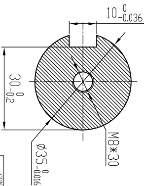
B-B (2:1)
