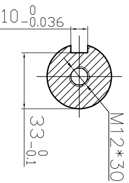
A-A(2:1)
