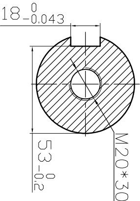
A-A(2:1)
