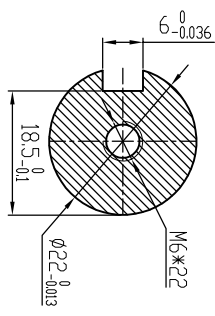
B-B (2:1)
