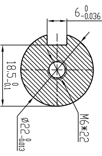
B-B (2:1)
