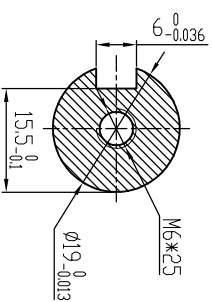
B-B (2:1)
