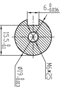
B-B (2:1)
