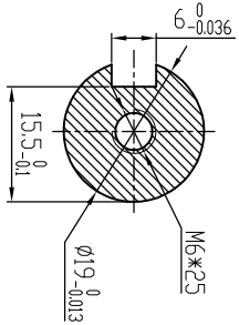
B-B (2:1)
