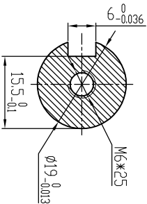
B-B (2:1)
