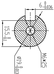
B-B (2:1)
