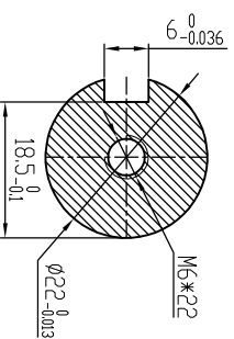
B-B (2:1)
