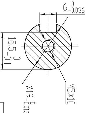
B-B (2:1)
